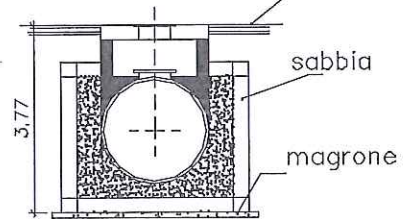
SEZIONE SEZIONE OR 002 quota str.le
